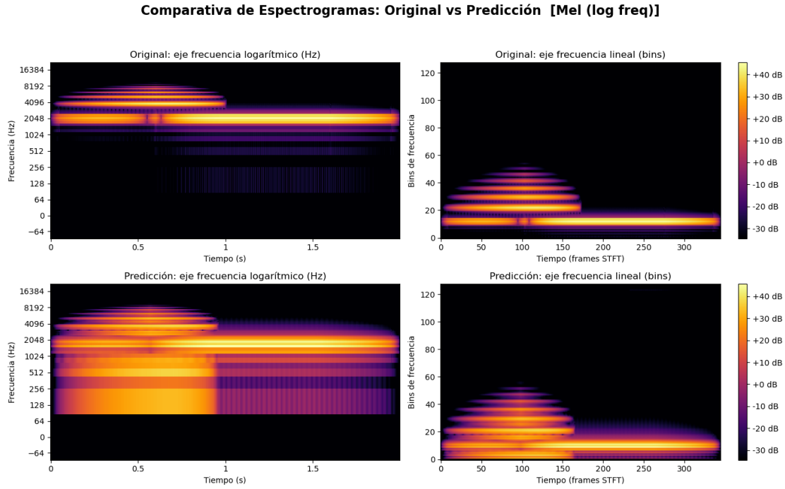
Figura 5.6: Espectrograma resultado de la predicción del audio de Benchmark: pad_lento .
