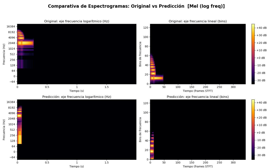
Figura 5.9: Espectrograma resultado de la predicción del audio de Benchmark: percusivo .
