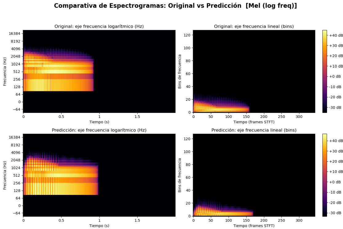
Figura 5.5: Espectrograma resultado de la predicción del audio de Benchmark: muy_bajo .
