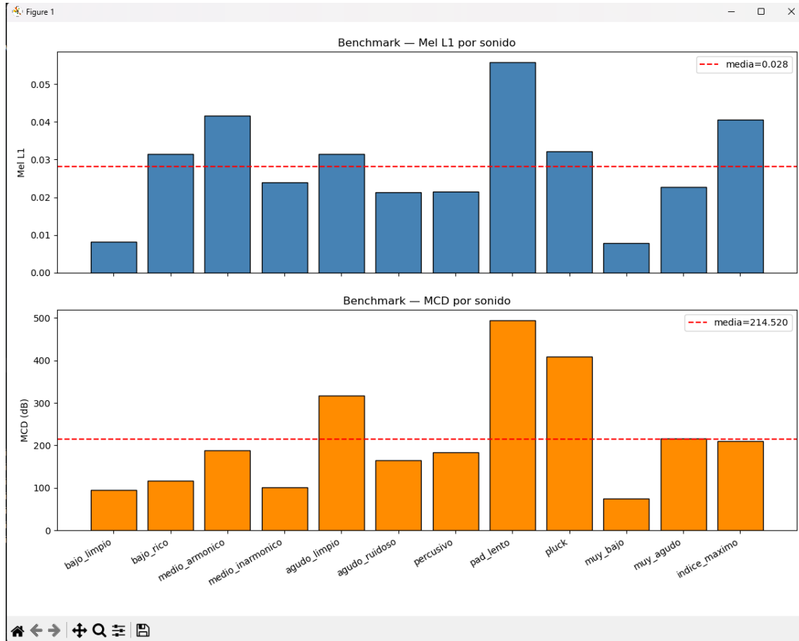
Figura 5.4: Gráfico obtenido en la evaluación de P2 mediante benchmark .
