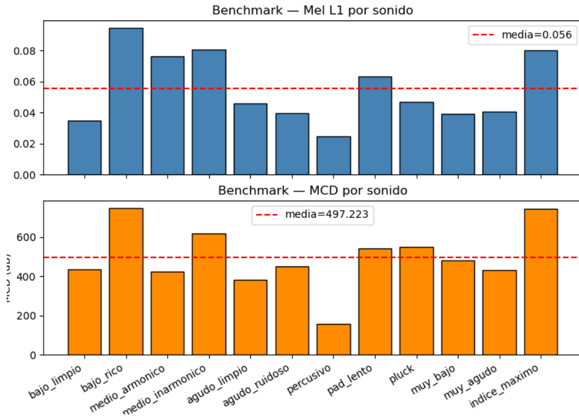
Figura 5.8: Gráfico obtenido en la evaluación de P4 mediante benchmark .
