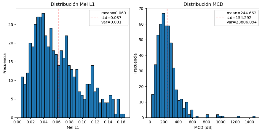
Figura 5.3: Graficas que muestran los resultados de evaluar el conjunto de tests sobre el modelo P2 con las métricas Mel L1 y MCD.
